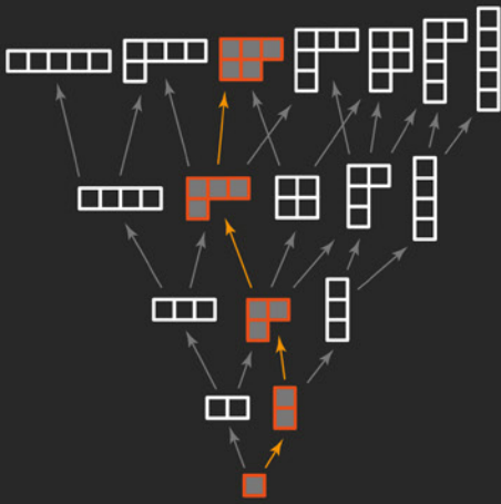
ENUMERATION
